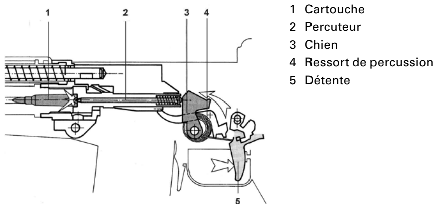
Figure 15: Départ du coup
