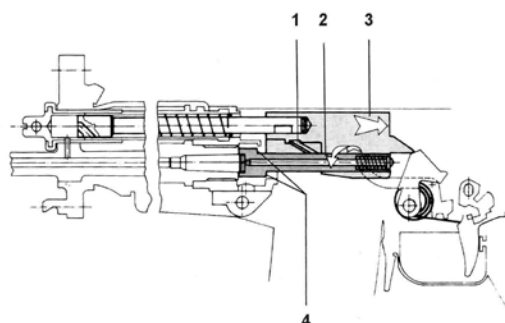
Figure 17: Déverrouillage de la culasse
