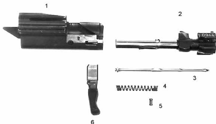
Figure 4: Culasse démontée
