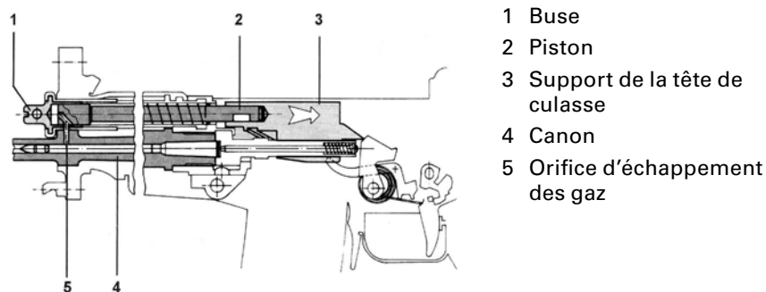
Figure 16: Recul du support de la tête de culasse
