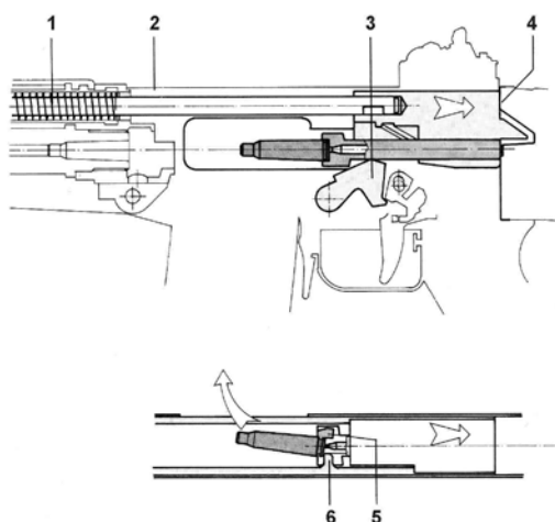
Figure 18: Recul de la culasse et éjection de la douille
